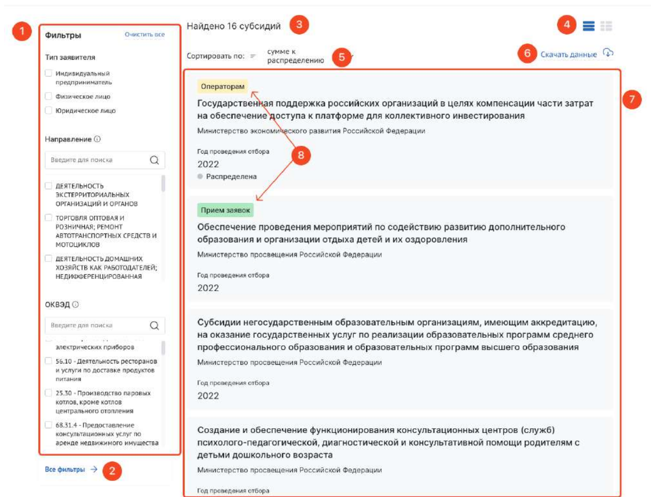
Рисунок 27. Страница «Навигатор», открытая на вкладке «Субсидии»
